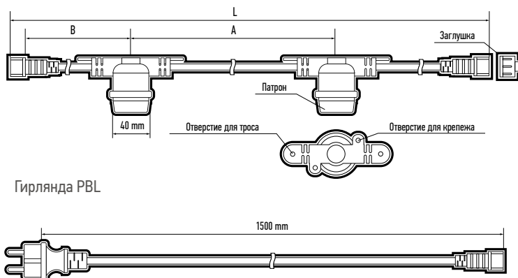
Сетевой шнур
