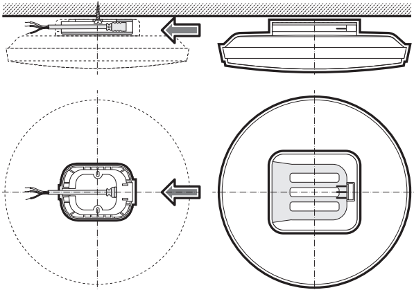
Рис. 2 Крепление монтажной рамки с сетевым коннектором к потолку
