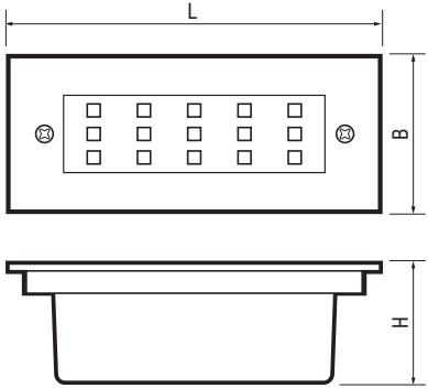
Рис.1 Светильник PWS/R
